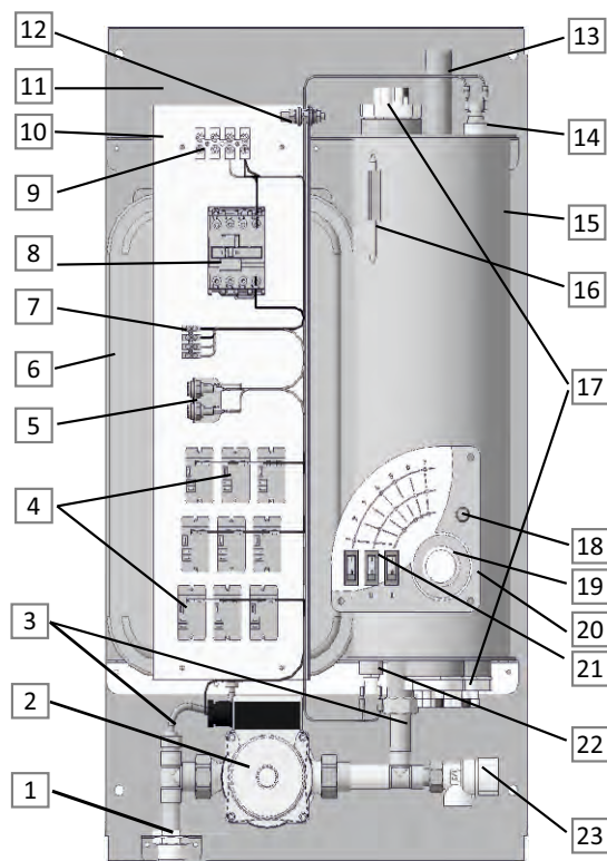
Устройство прибора
